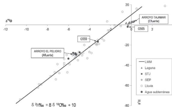
Figura 7. Contenido isotópico ( \delta^{18}\text{O} y \delta^2\text{H} ) en el agua subterránea, arroyos, laguna y agua de lluvia. Isotopic content ( \delta^{18}\text{O} and \delta^2\text{H} ) in the groundwater, streams, wetland, and rainfall.
